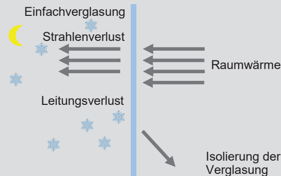
Einfachverglasung im Winter
